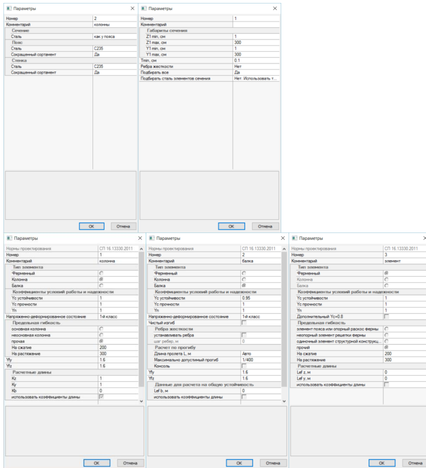
Рис 6. Заданные параметры материалов элементам схемы
